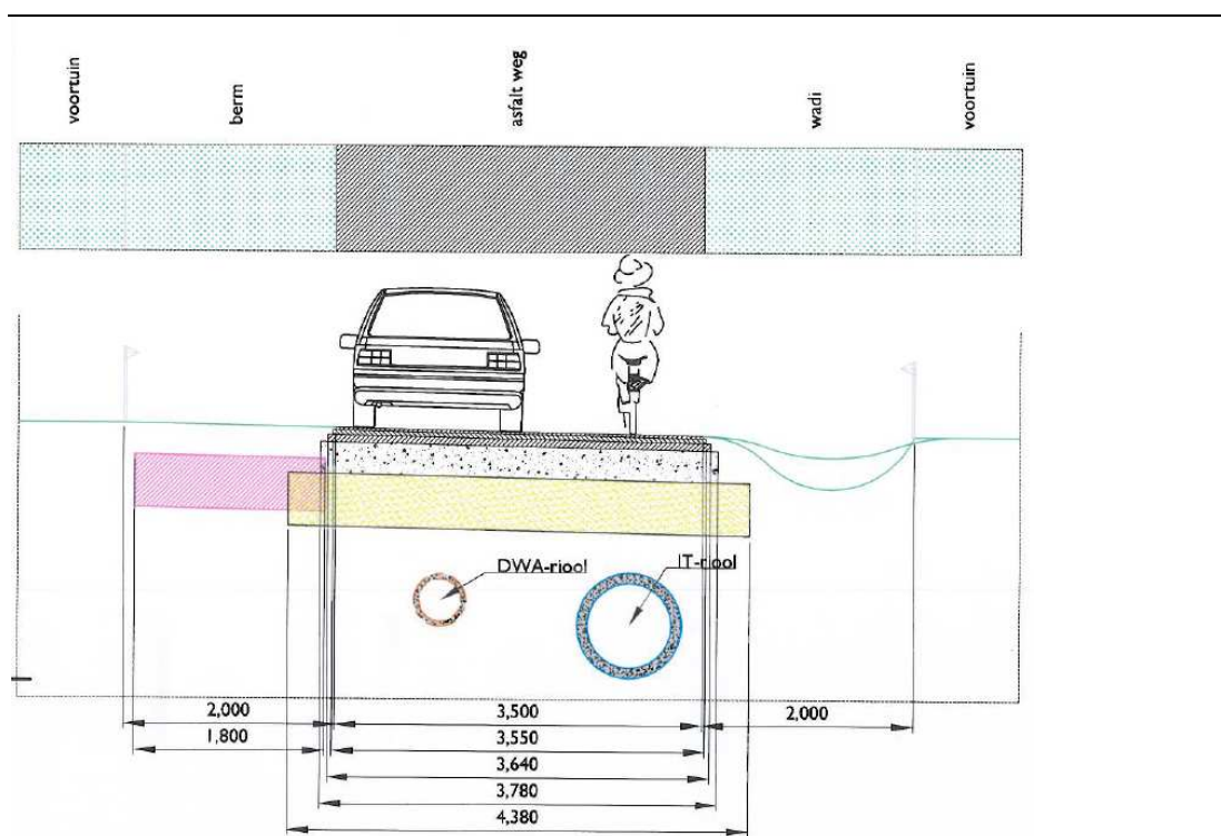
Figuur 3.1 Profiel greppels plangebied bij asfaltwegen
