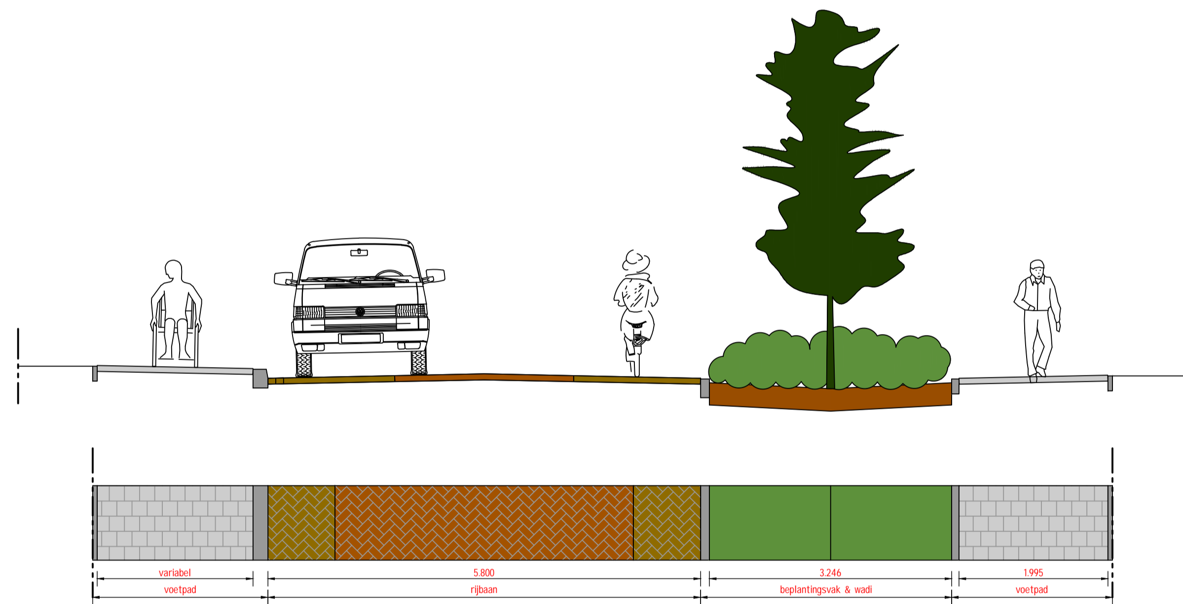
principedoorsnede/ bovenaanzicht Doetinchemseweg (t.h.v. huisnr. 14) schaal 1:50
