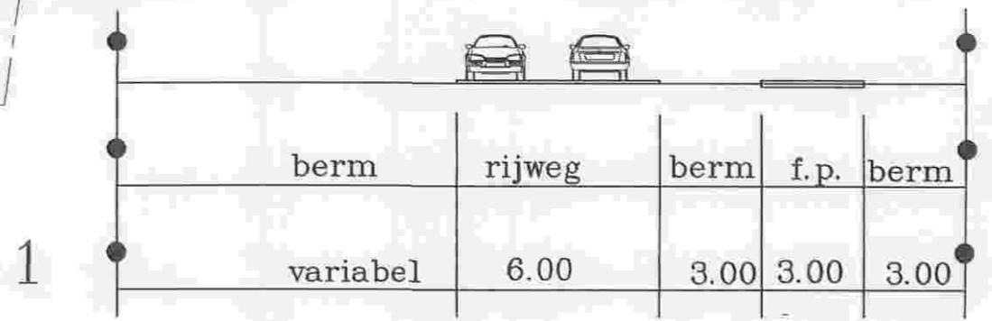
DWARSPROFIEL SCHAAL 1:200
