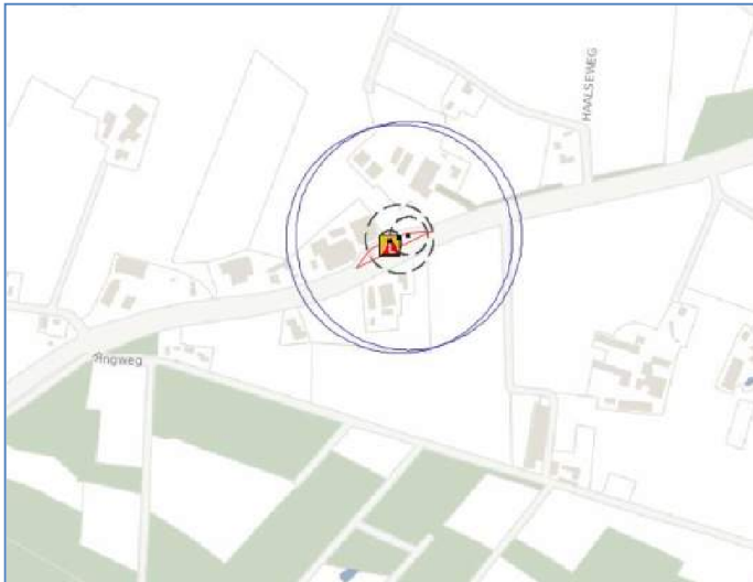
Afbeelding 2.1: Risikocontouren LPG-tankstation
