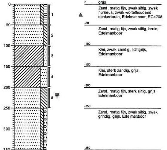
Boring: 342 Datum: 29-09-2005
