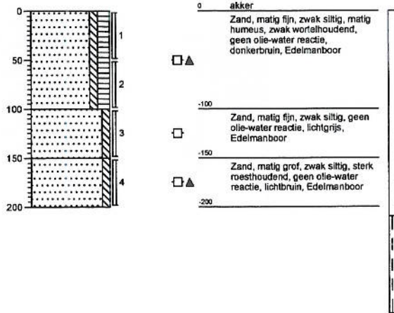
Boring: 064 Datum: 05-10-2005
