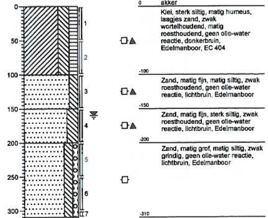
Boring: 065 Datum: 05-10-2005
