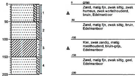
Boring: 333 Datum: 29-09-2005
