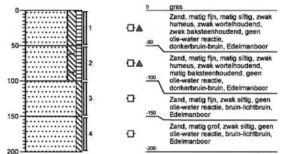
Boring: 241 Datum: 03-10-2005
