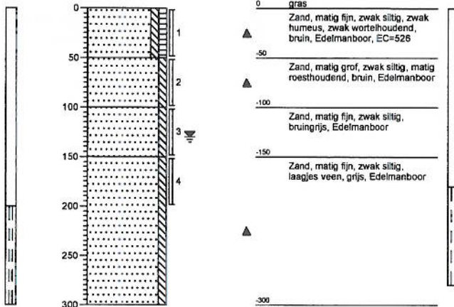
Boring: 339 Datum: 29-09-2005
