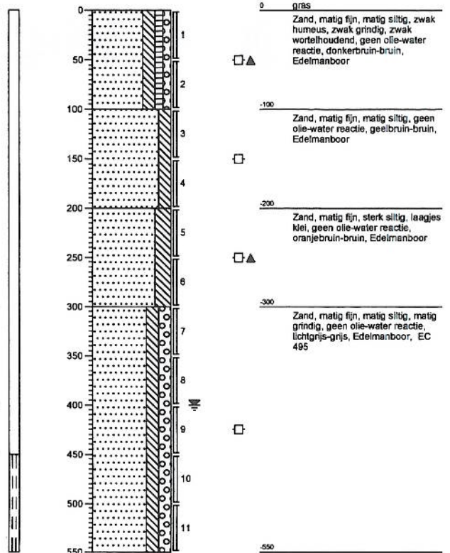
Boring: 241 Datum: 03-10-2005
