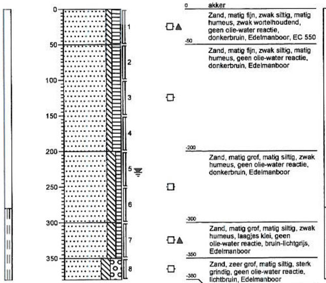
Boring: 066 Datum: 05-10-2005
