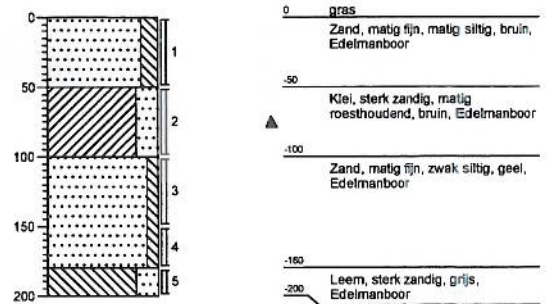
Boring: 304 Datum: 30-09-2005
