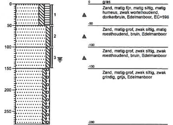
Boring: 340 Datum: 29-09-2005
