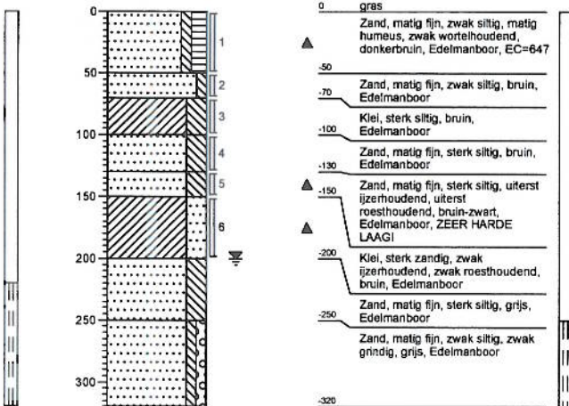
Boring: 341 Datum: 29-09-2005
