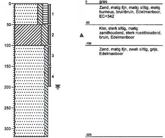
Boring: 332 Datum: 29-09-2005
