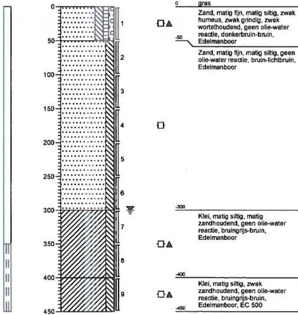
Boring: 238 Datum: 03-10-2005
