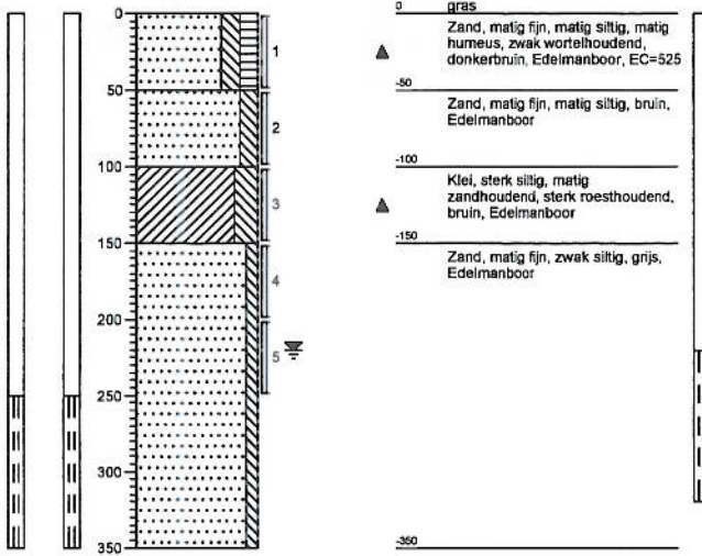
Boring: 331 Datum: 29-09-2005
