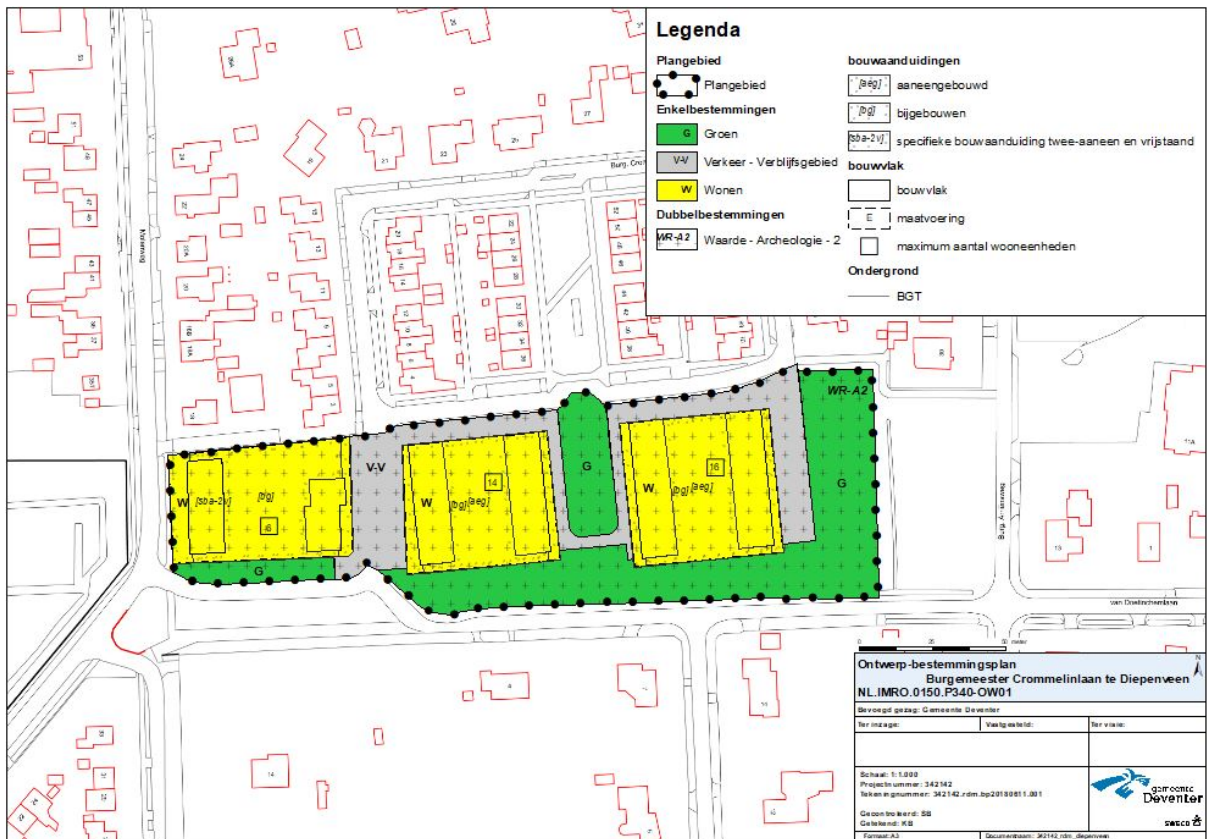
Afbeelding 5.1 - Planverbeelding
