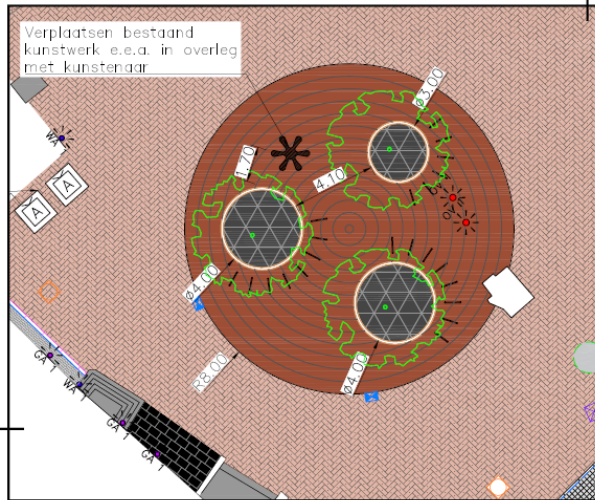
Huidige ontwerp
