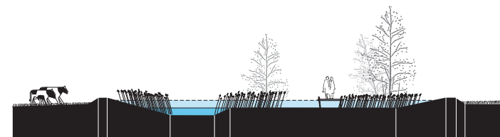
Profiel van de Zandwetering in het landbouwgebied
