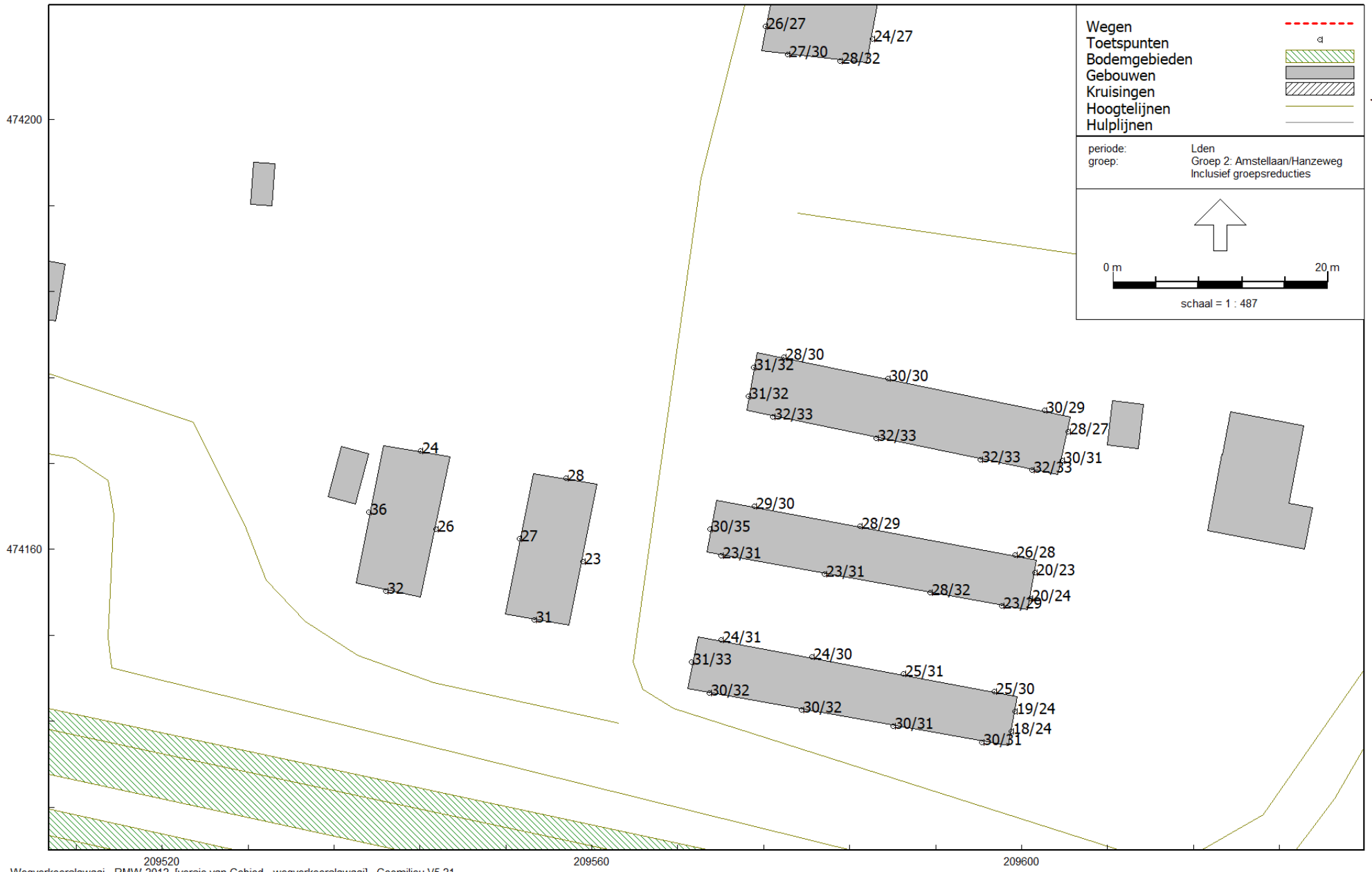
Wegverkeerslawaai - RMW-2012, [versie van Gebied - wegverkeerslawaai], Geomilieu V5.21
