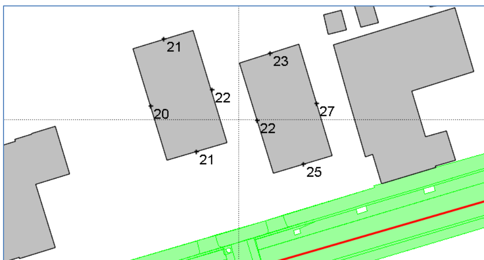
Figuur 4 Hoogst berekende geluidbelasting vanwege de Worp inclusief aftrek conform artikel 110g Wgh
