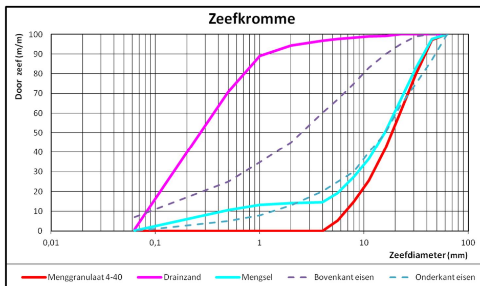
Figuur 27: Zeefkromme
