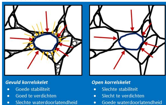
Figuur 19: Eigenschappen korrelskelet
