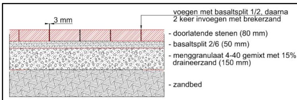
Figuur 25: Dwarsprofiel van het geadviseerde ontwerp
