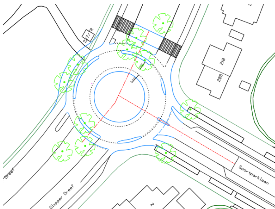
Schetssteking rotonde kruising Glipper Dreef – Sportparklaan
