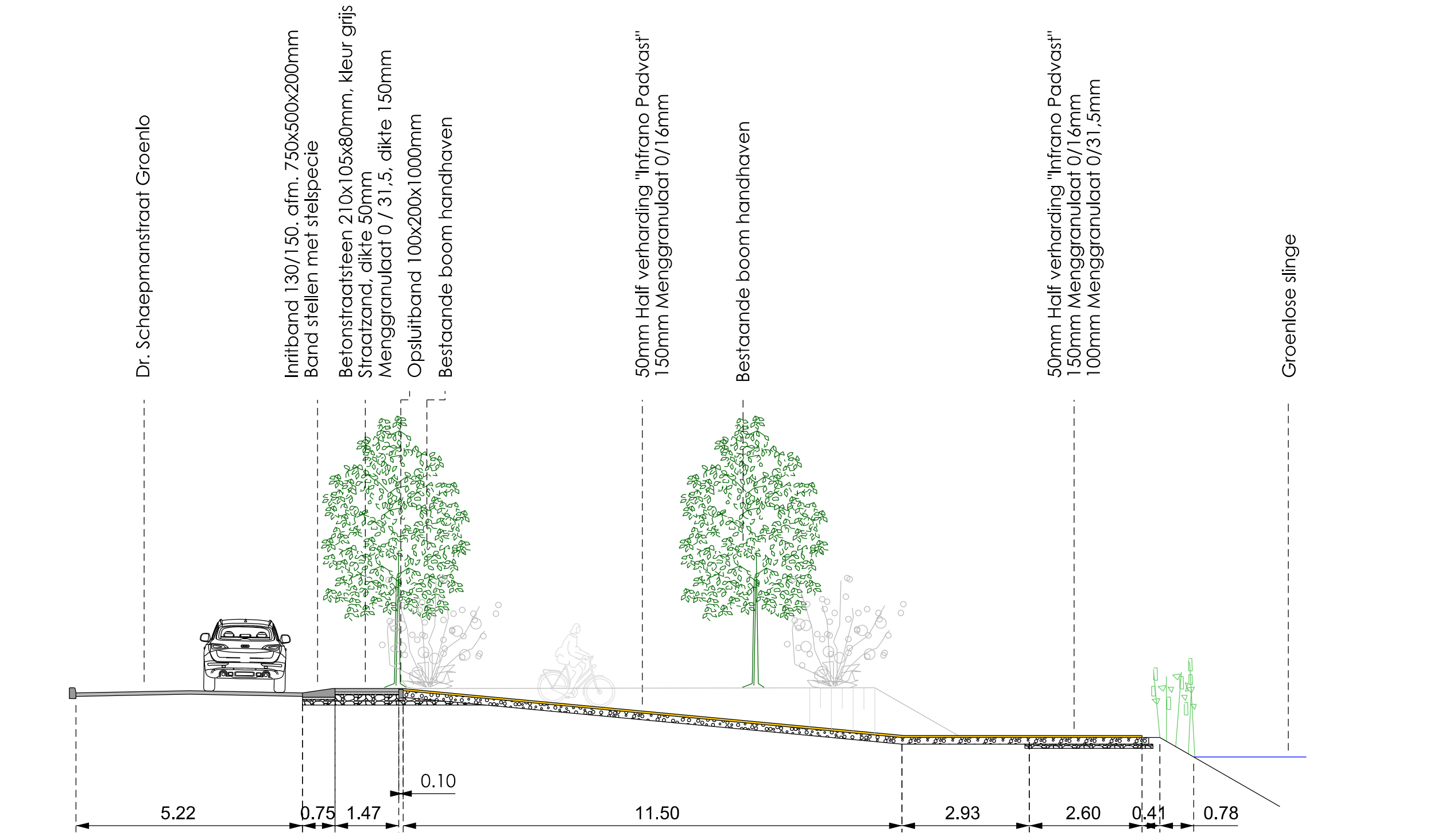
Dwarsprofiel A - A' Nieuwe situatie (schaal 1:100)
