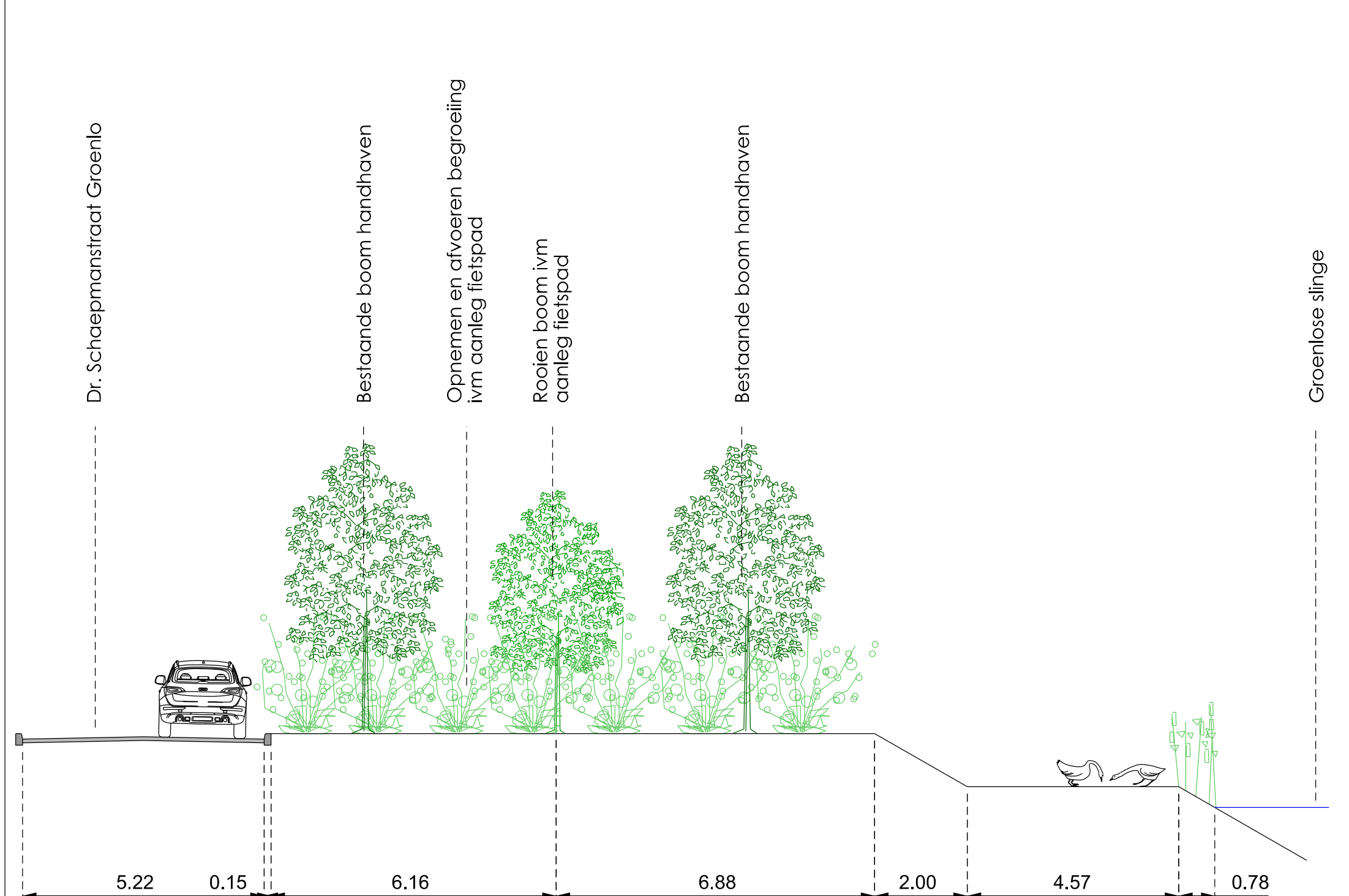
Dwarsprofiel A - A' Bestaande situatie (schaal 1:100)
