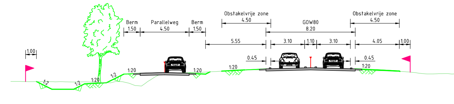
Dwarsprofiel A-A, GOW 80km/h met parallelweg Schaal 1:200
