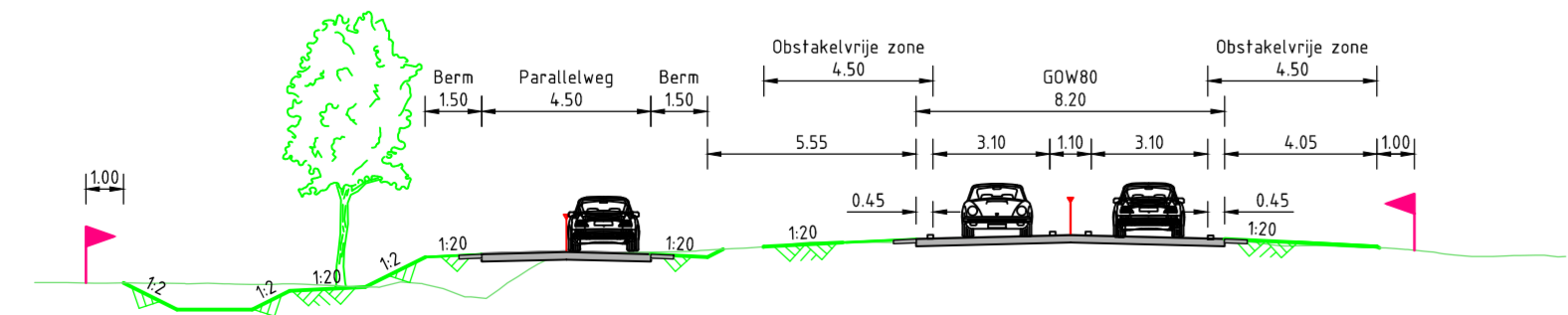
Dwarsprofiel A-A, GOW 80km/h met parallelweg Schaal 1:200
