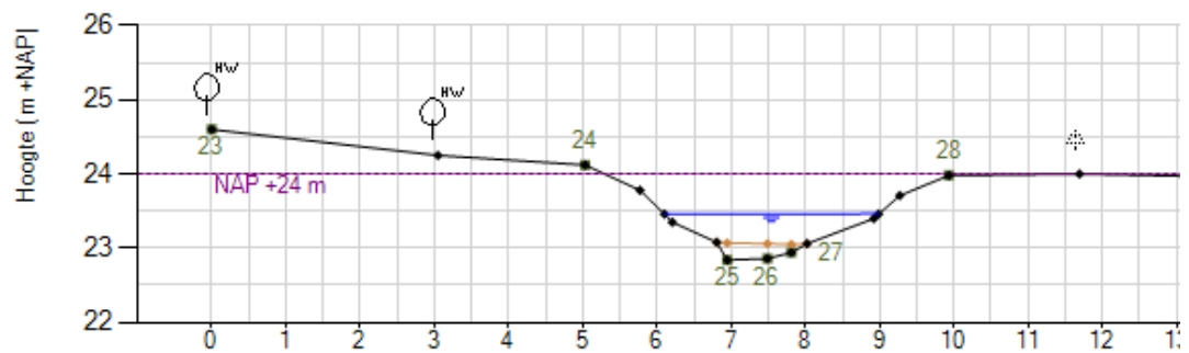
Figuur 1 Leggerprofiel
