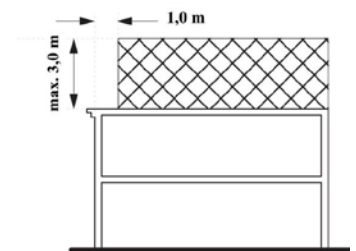
Doorsnede dakopbouw op plat dak
